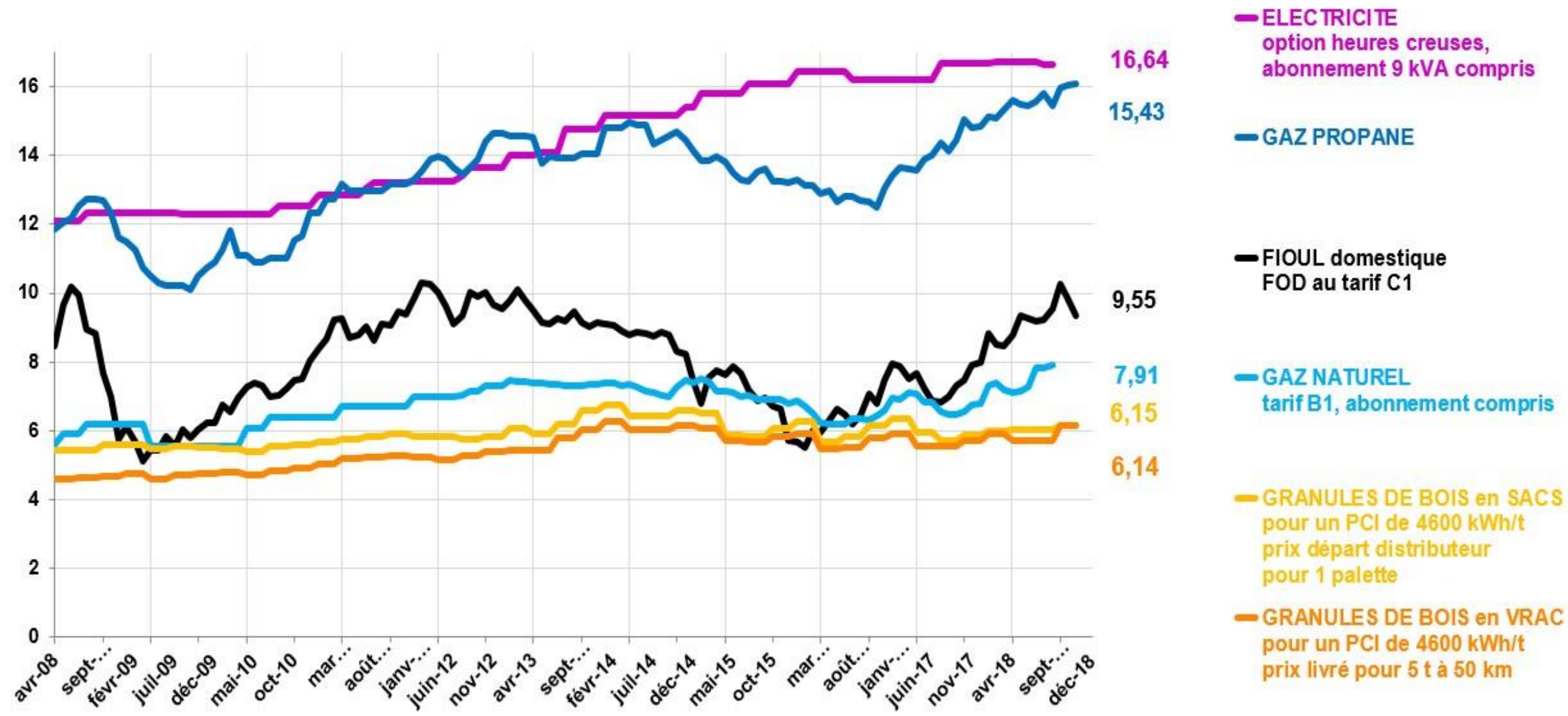
Evolution du coût des énergies en centimes d'euros TTC/kWh PCI pour un usage en chauffage principal - source: SOeS - CEEB / Propellet France - Décembre 2018
